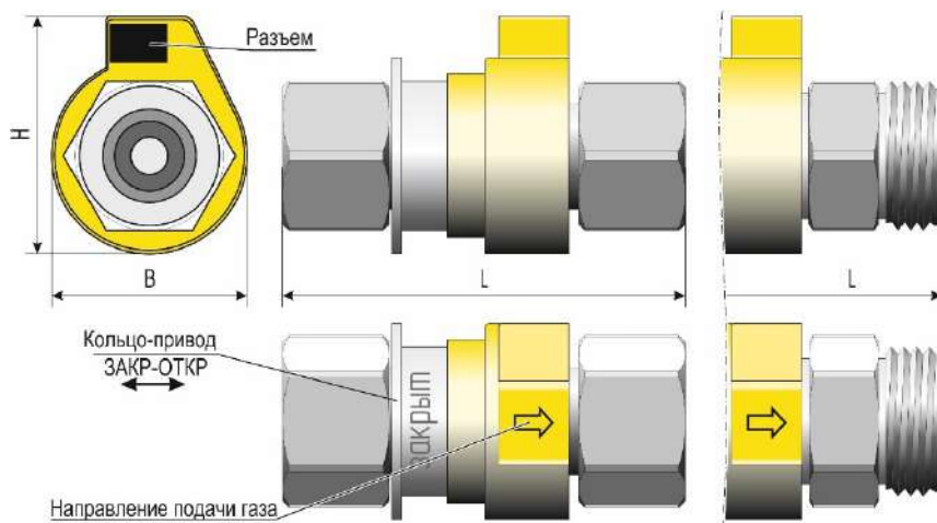
а) исполнения «муфта», «накидная гайка» б) исполнение «штуцер» Рисунок 1 – Внешний вид клапана
